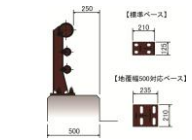
ワイドベース&地覆巾 500対応両用タイプ
